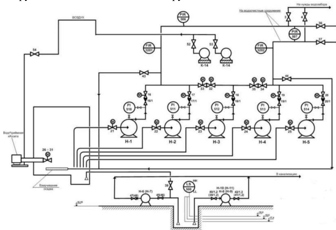
Рисунок 5. Технологическая схема Епанчинского водозабора.
