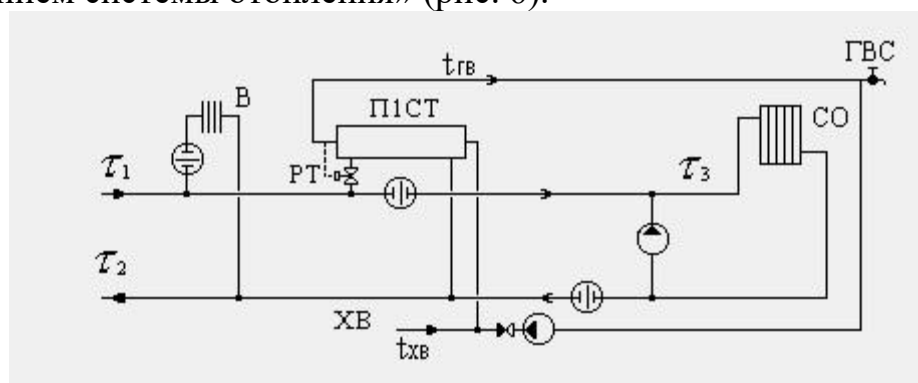
Рисунок 6. Схема технологического присоединения потребителей к ЦТП (схема № 23 в Zulu Termo)
