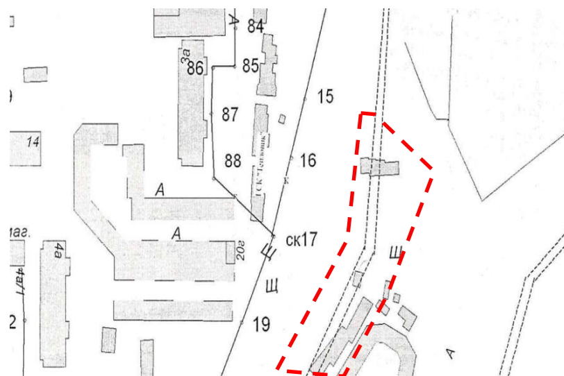
Рисунок 17. Сети канализации диаметром \varnothing 1000 мм, необходимые к выносу
