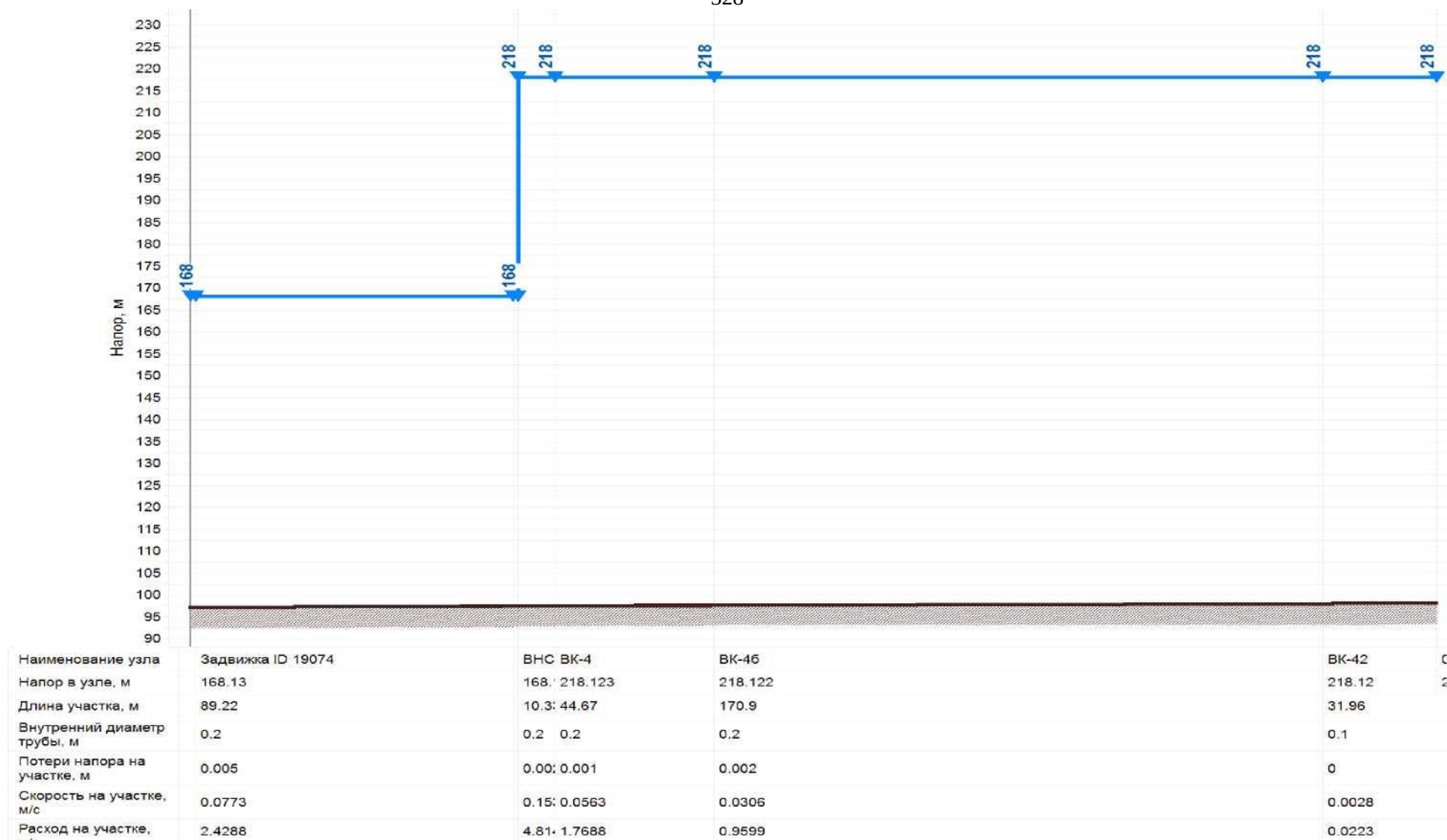
Рисунок 11. Пьезометрический график водопроводной сети от города Тобольска от ВК-19а/ПГ до потребителя по адресу 6-й микрорайон, 1 (Пример)
