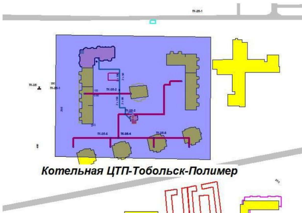
Рисунок 15. Перспективная схема зон действия централизованной системы горячего водоснабжения с привязкой к топографической основе города Тобольска (7а мкр., ЦТП-Тобольск-Полимер)
