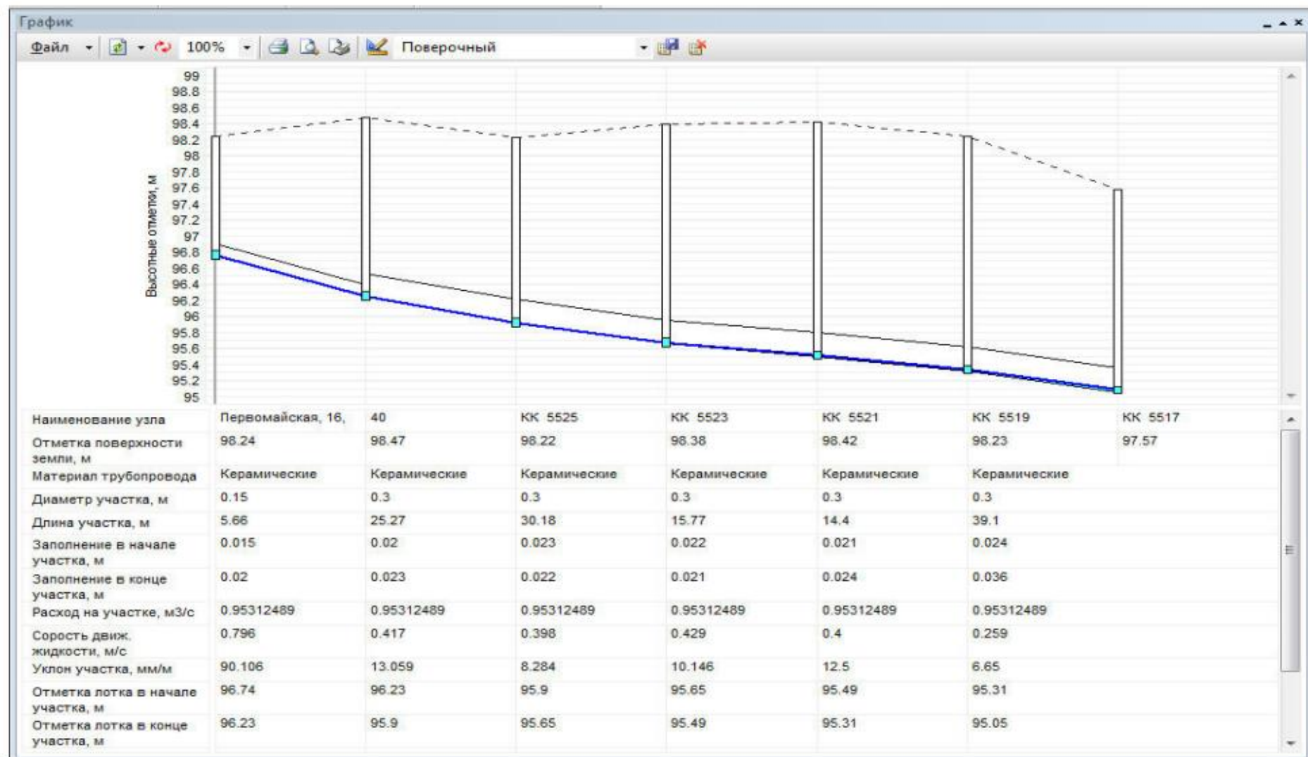
Рисунок 10. Продольный профиль канализационной сети города Тобольска от ул. Первомайской, 16 до КК 5517 (Пример)
