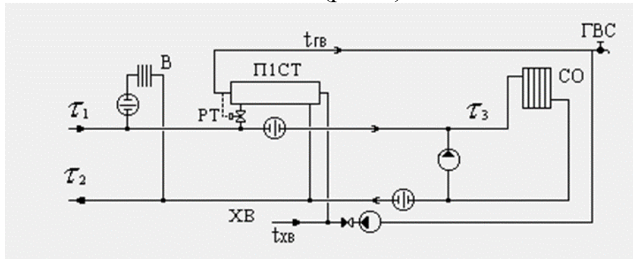
Рисунок 5. Схема технологического присоединения потребителей к ЦТП (схема № 23 в Zulu Termo)
