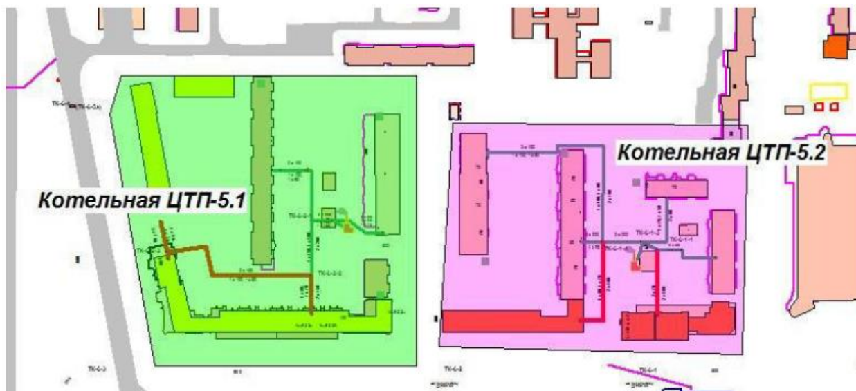
Рисунок 16. Перспективная схема зон действия централизованной системы горячего водоснабжения с привязкой к топографической основе города Тобольска (7 мкр., ЦТП-5.1, 5.2)
