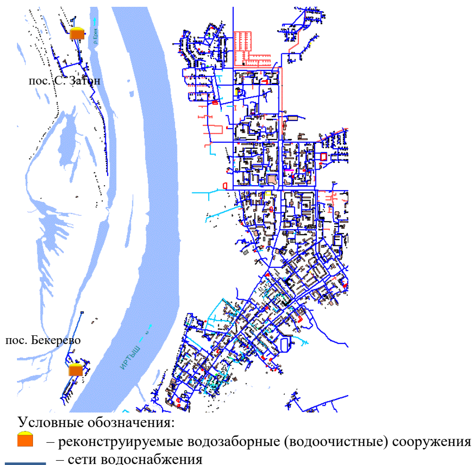
Рисунок 10. Перспективное размещения объектов системы водоснабжения ТО Левобережье (вариант 1)
