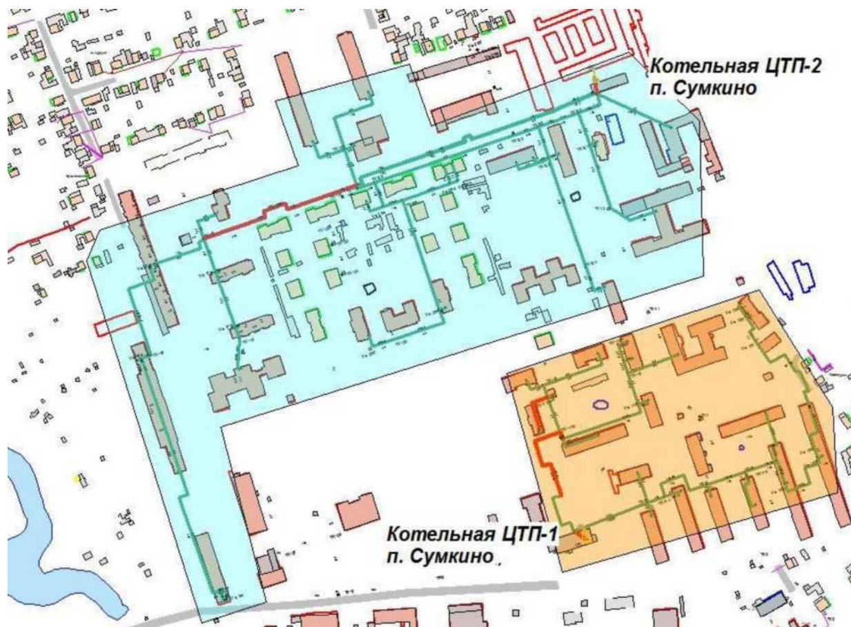
Рисунок 17. Перспективная схема зон действия централизованной системы горячего водоснабжения с привязкой к топографической основе города Тобольска (пос. Сумкино, ЦТП-1, 2)
