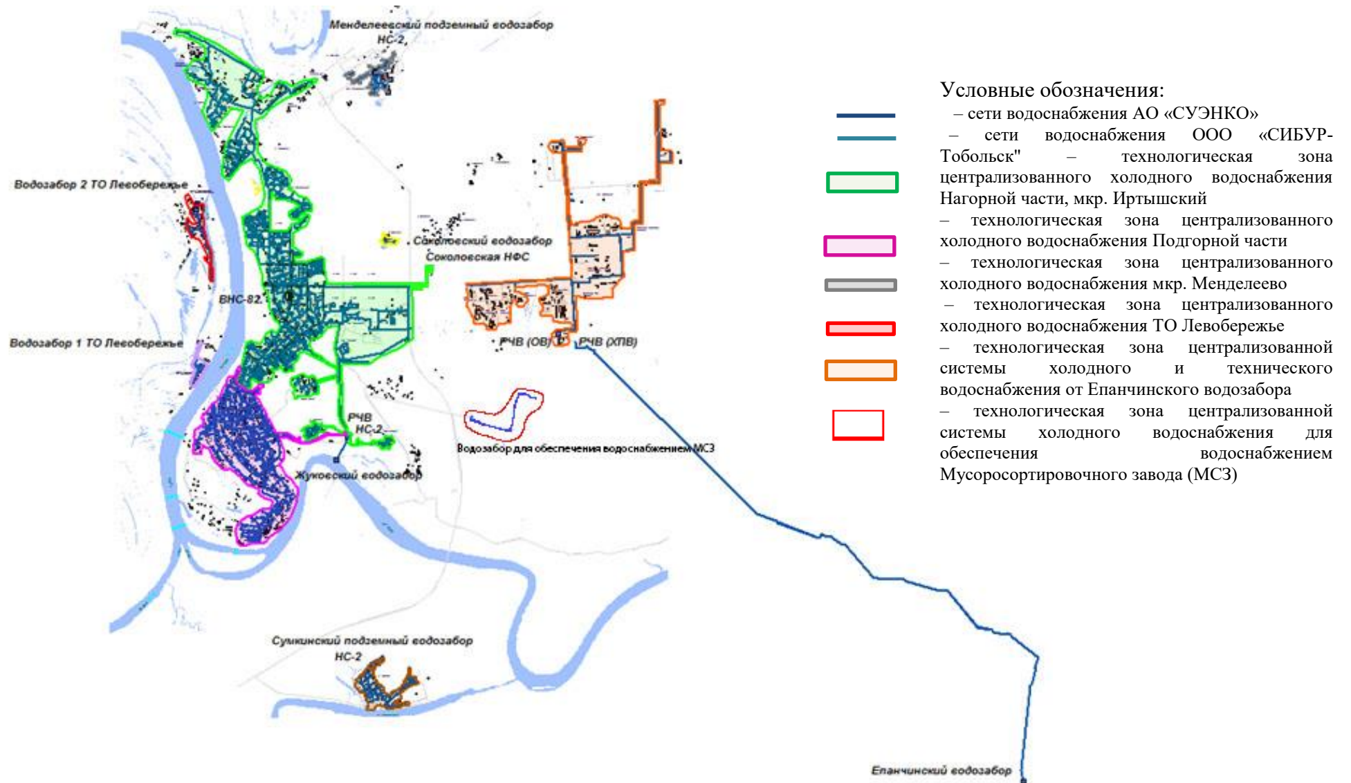
Рисунок 2. Технологические зоны централизованных систем холодного водоснабжения города Тобольска
