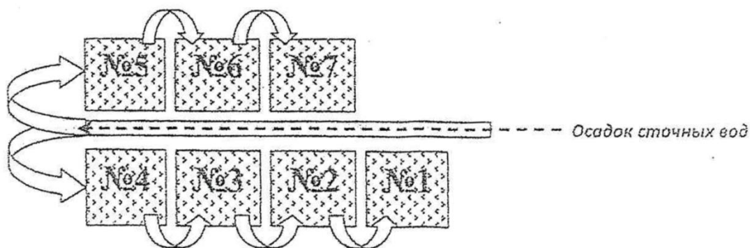
Рисунок 28. Схема расположения иловых карт
