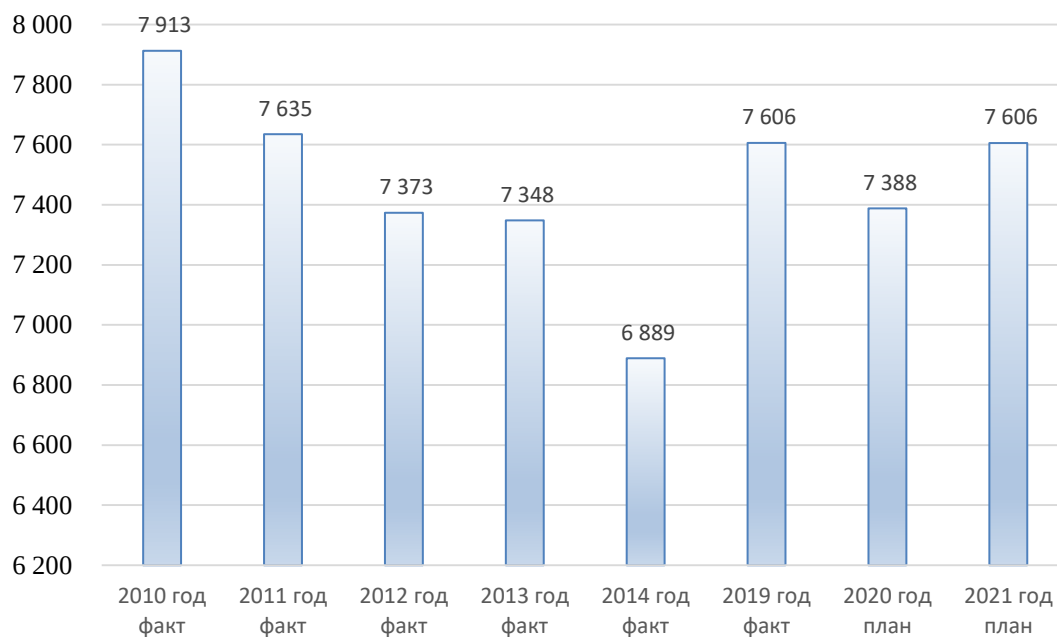
Рисунок 23. Динамика поступления сточных вод в централизованную систему водоотведения по городу Тобольску тыс. м³
