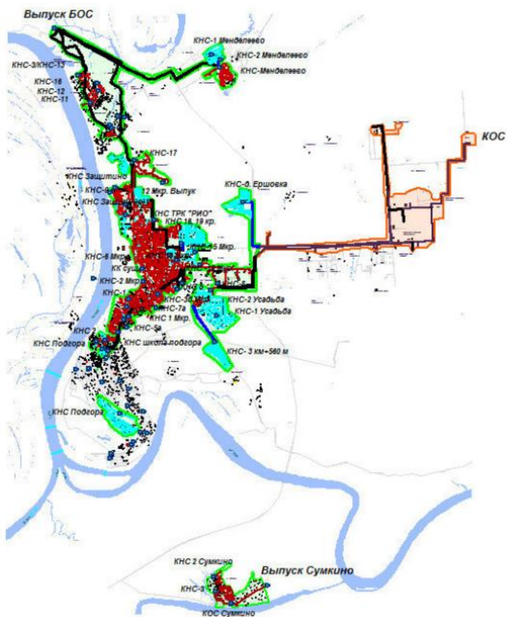
Рисунок 14. Перспективная схема централизованной системы водоотведения города Тобольска с привязкой к топографической основе города
