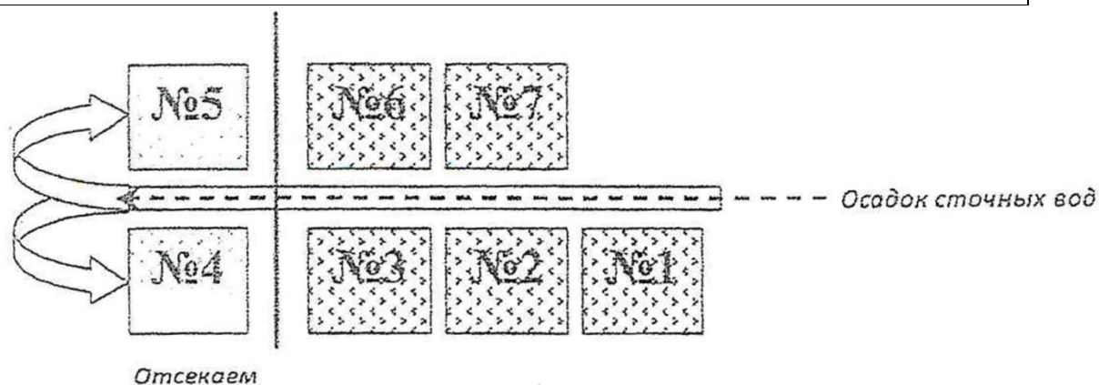
Рисунок 29. Схема очистки иловых карт
