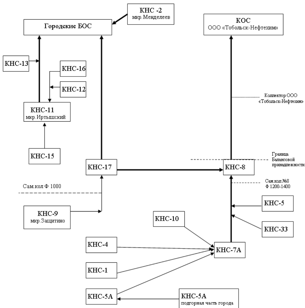
Рисунок 22. Организационная схема перекачки стоков города Тобольска
