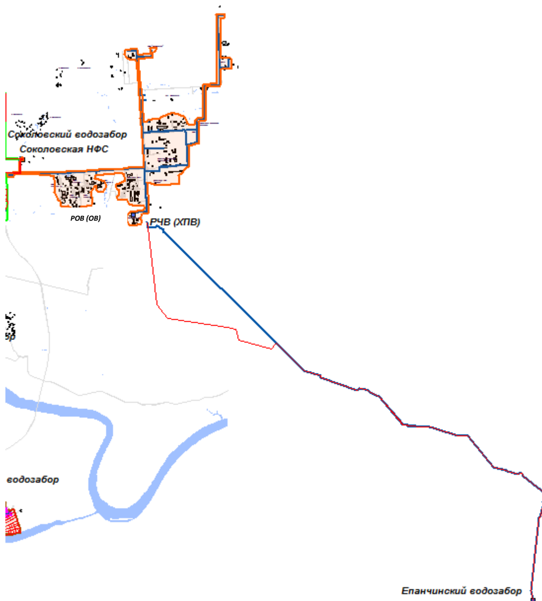
Рисунок 16. Маршруты прохождения трассы по водоводу от Епанчинского водозабора до ВОС
