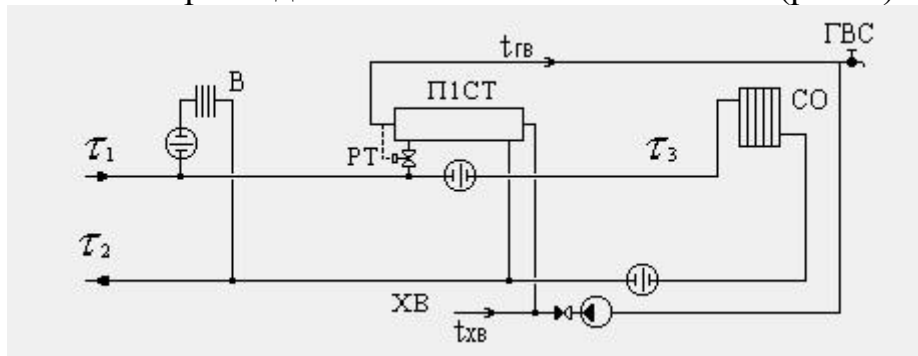
Рисунок 6. Схема технологического присоединения потребителей мкр. Иртышский (схема № 28 в Zulu Termo)
