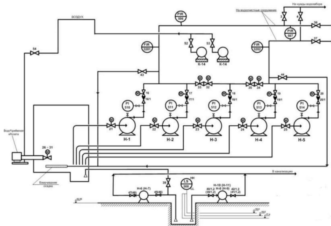
Рисунок 4. Технологическая схема Епанчинского водозабора.
