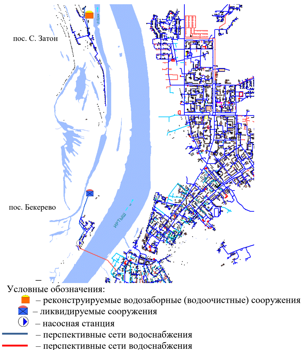
Рисунок 11. Развитие системы водоснабжения ТО Левобережье (вариант 2)
