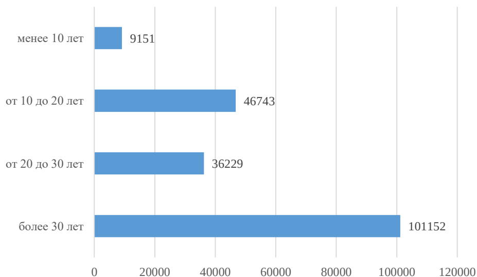
Рисунок 21. - Данные по протяженности, м, и сроку службы канализационных сетей
