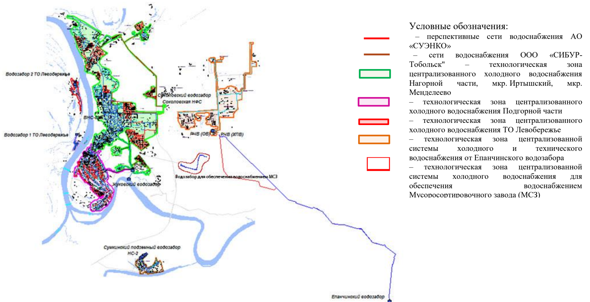
Рисунок 8. Зоны с централизованными системами водоснабжения города Тобольска на перспективу до 2032 года (с выделением технологических зон водоснабжения)
