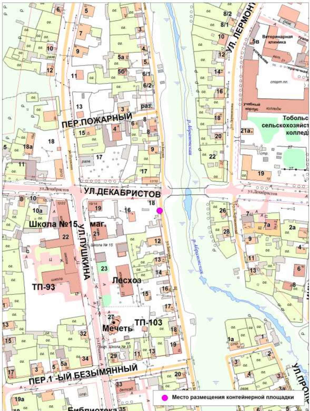
Схема размещения контейнерной площадки по адресу: Тюменская область, г.Тобольск, ул.Декабристов/ул.Басова, 18/11, М 1:2000
