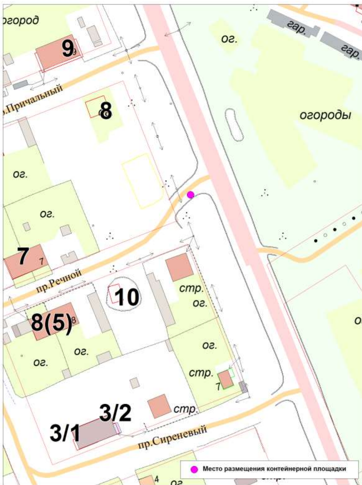
Схема размещения контейнерной площадки по адресу: Тюменская область, г.Тобольск, мкр. Иртышский, пересечение ул.Портовая и пр.Речной М 1:1000
