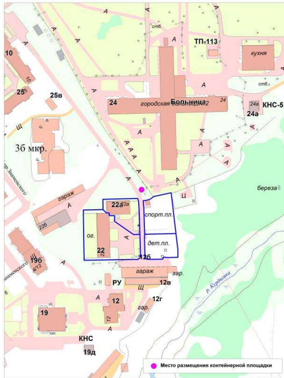
Схема размещения контейнерной площадки по адресу: Тюменская область, г.Тобольск, 36 мкр., д.22, 22а М 1:1500
