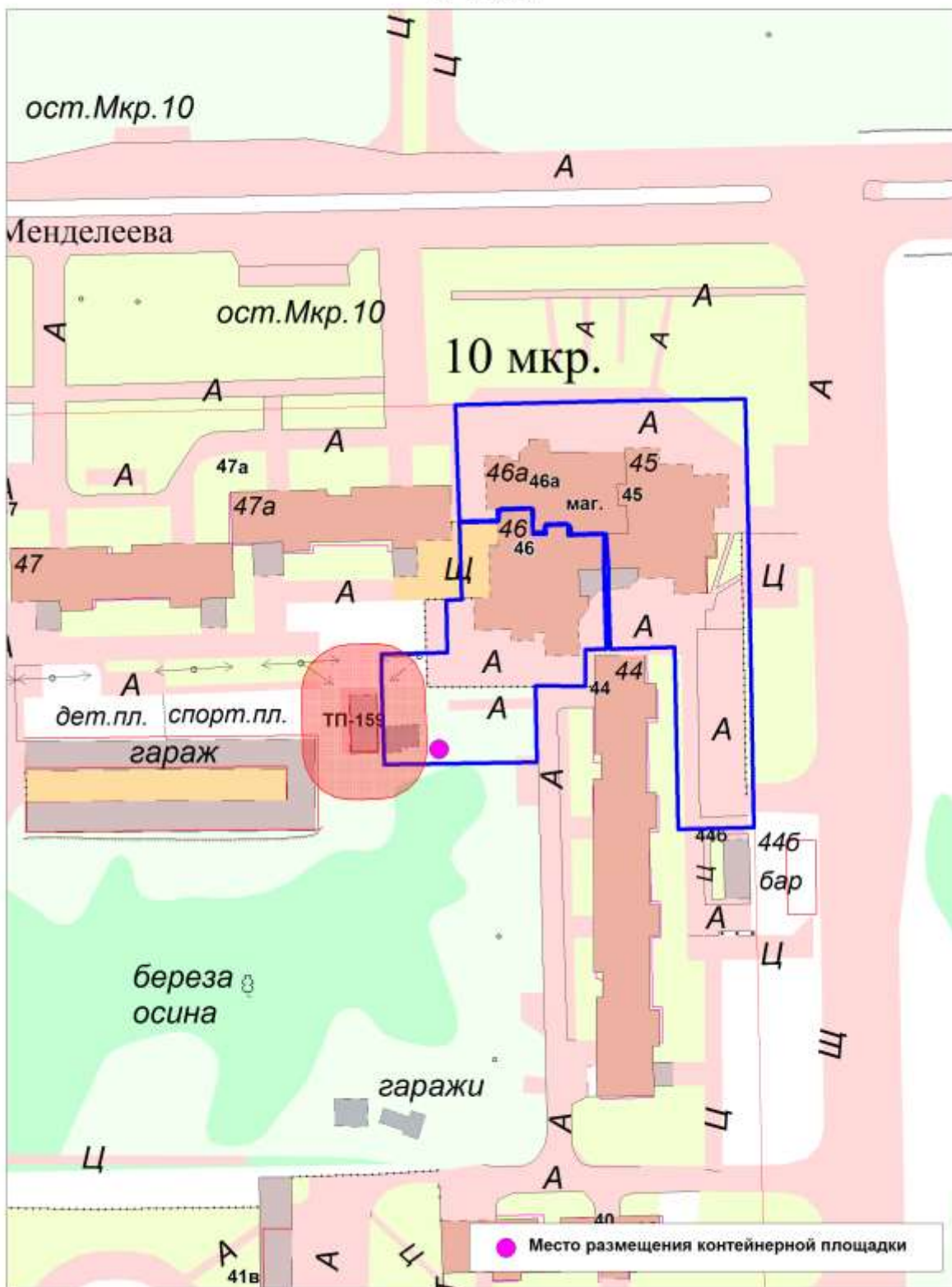
Схема размещения контейнерной площадки по адресу: Тюменская область, г.Тобольск, 10 мкр., стр.46а М 1:1000
