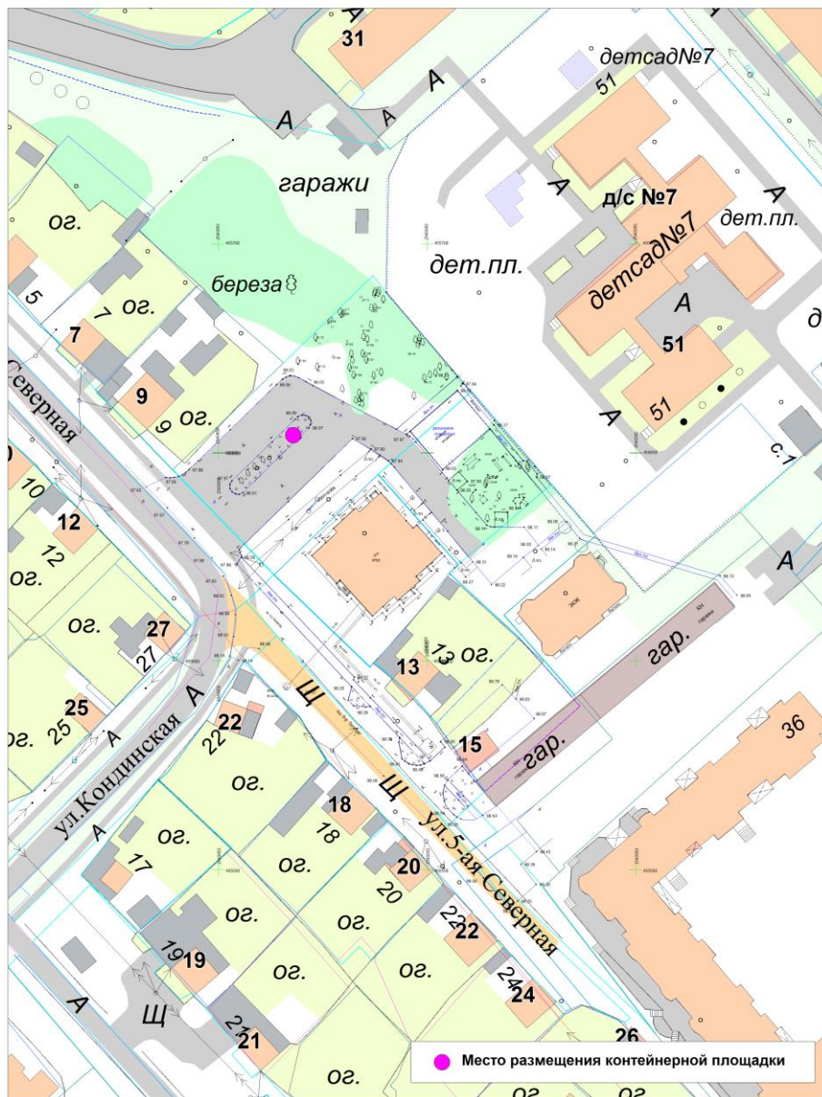
Схема размещения контейнерной площадки по адресу: Тюменская область, г.Тобольск, 4 мкр., д.366 М 1:1000
