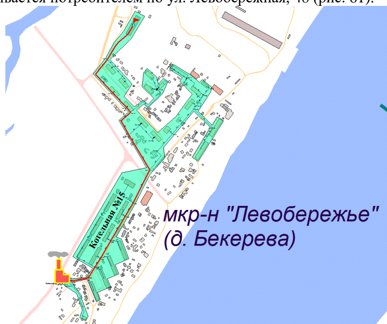
Рисунок 63. Трассировка участка тепловой сети от камеры «Вывод - Котельная № 15» до потребителя по ул. Левобережная, 48
