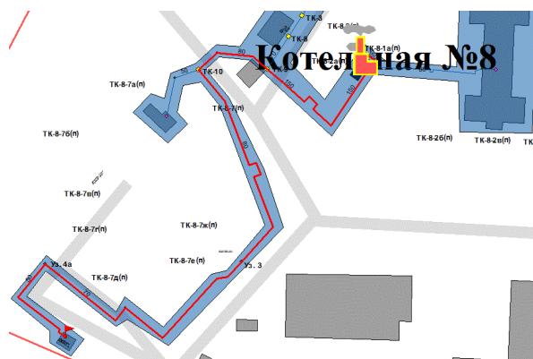
Рисунок 33. Трассировка участка тепловой сети от камеры «Вывод Котельная № 8» до потребителя по ул. Ершова, 2
