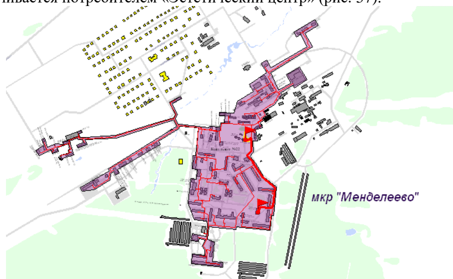
Рисунок 59. Трассировка участка тепловой сети от камеры «Вывод - Котельная № 22» до потребителя «Эстетический центр»
