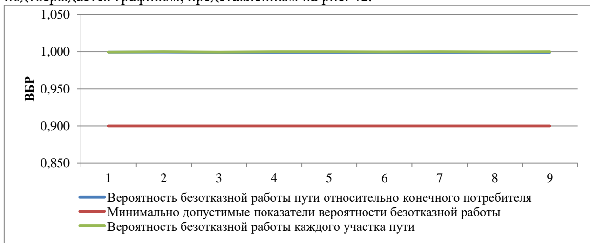
Рисунок 44. ВБР относительно участка тепловой сети от камеры «Вывод Котельная № 17» до потребителя «Пединститут, столовая»
