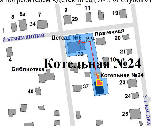
Рисунок 47. Трассировка участка тепловой сети от камеры «Вывод - Котельная № 24» до потребителя «Детский сад № 5 «Голубок»
