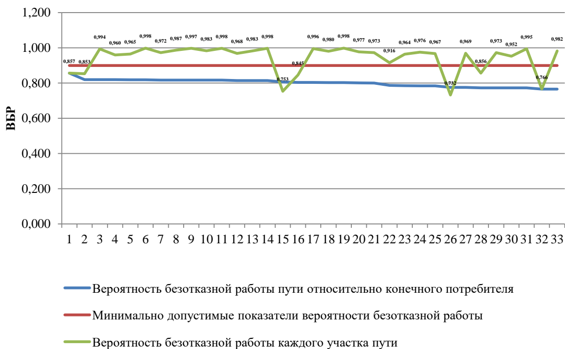
Рисунок 26. Вероятности безотказной работы относительно участка тепловой сети от Тобольской ТЭС до Уз. А, Потребитель «Город»
