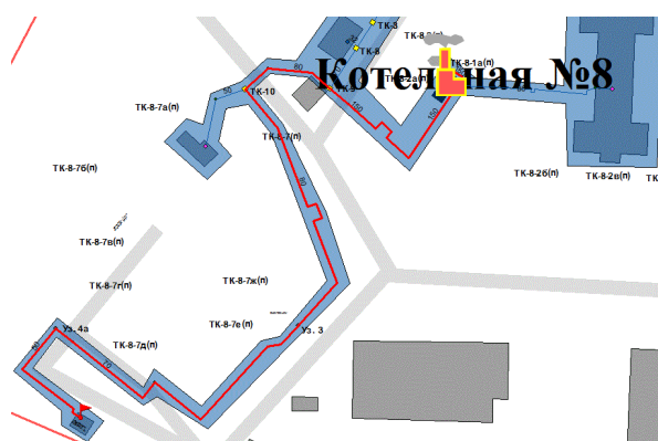
Рисунок 30. Трассировка участка тепловой сети от камеры «Вывод Котельная № 8» до потребителя по ул. Ершова, 2
