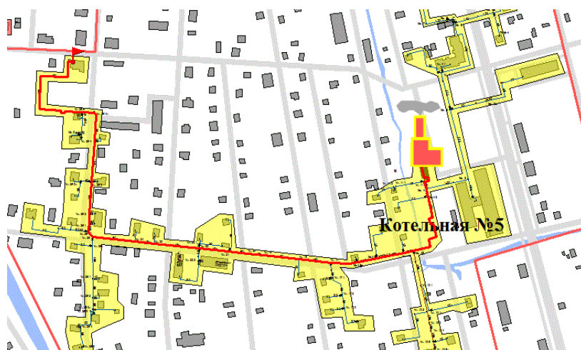
Рисунок 26. Трассировка участка тепловой сети от камеры «Вывод - Котельная № 5» до потребителя по ул. Семакова, 58
