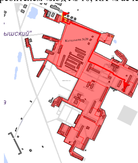
Рисунок 54. Трассировка участка тепловой сети от камеры «Вывод - Котельная № 20» до потребителя «Ж/д № 10, КХ «Расчет»
