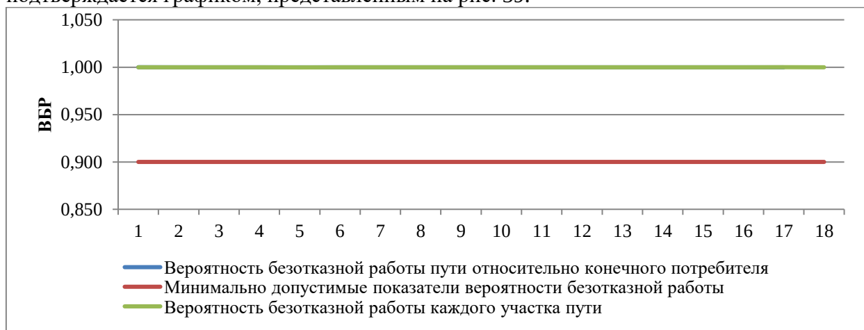
Рисунок 35. ВБР относительно участка тепловой сети от камеры «Вывод - Котельная № 12» до потребителя по ул. Гоголя, 41
