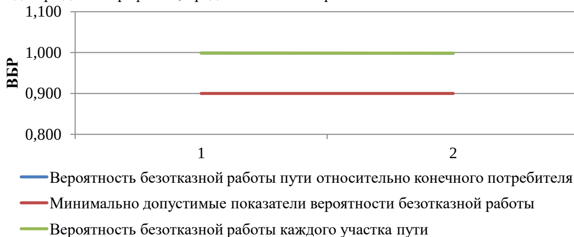
Рисунок 69. ВБР относительно участка тепловой сети от камеры «Вывод -Котельная № 2» до потребителя по ул. Октябрьская, 57
