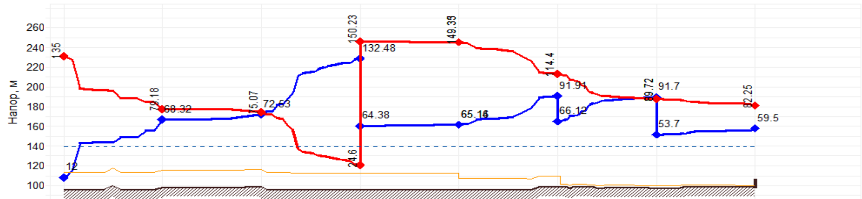
Пьезометрический график от «Тобольская ТЭЦ» до «Архив-2»
