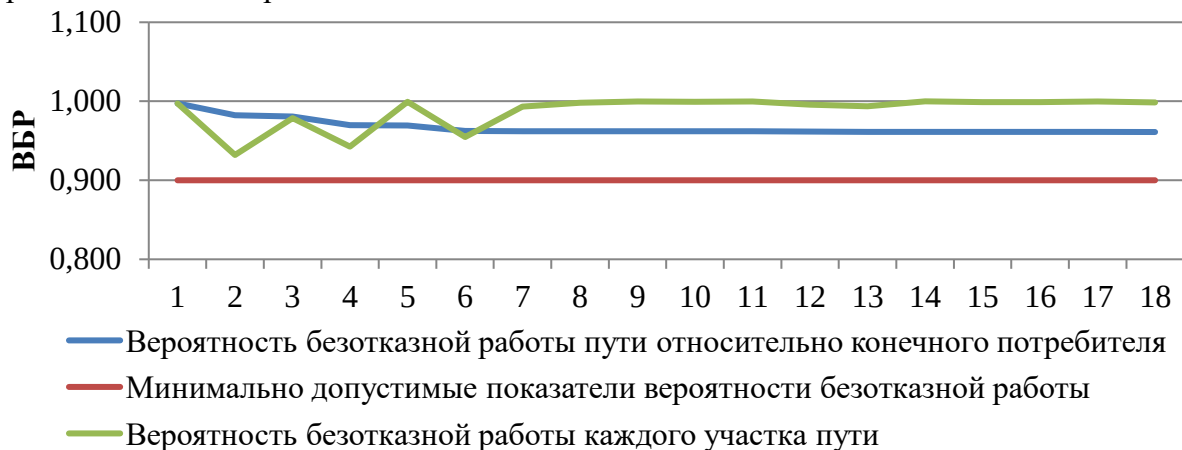
Рисунок 67. ВБР относительно участка тепловой сети от камеры «Вывод - Котельная № 11» до потребителя по ул. Водников, 3.
