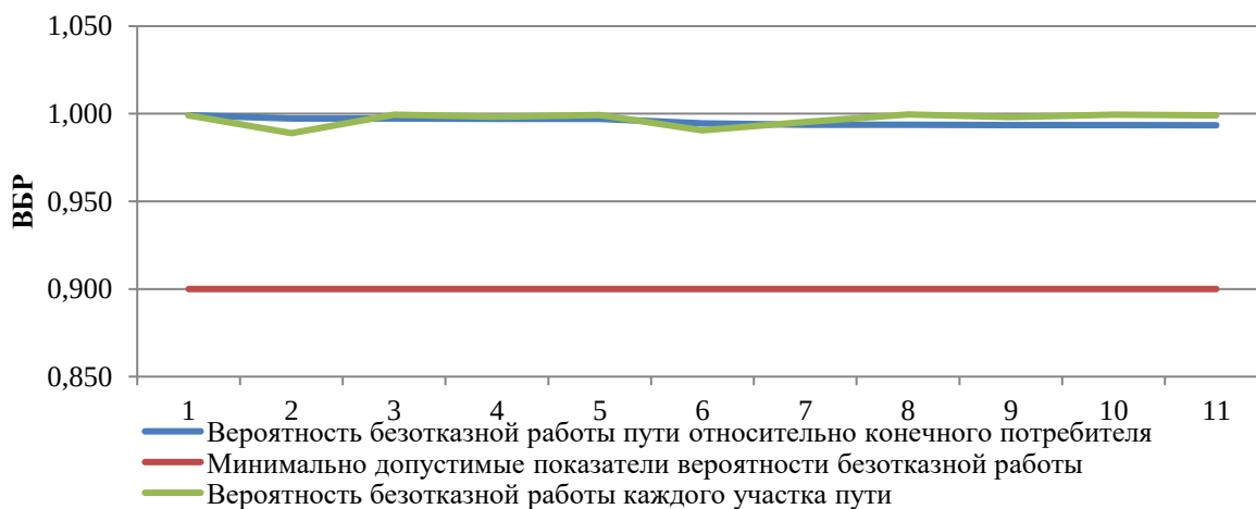
Рисунок 31. ВБР относительно участка тепловой сети от камеры «Вывод - Котельная № 8» до потребителя по ул. Ершова, 2
