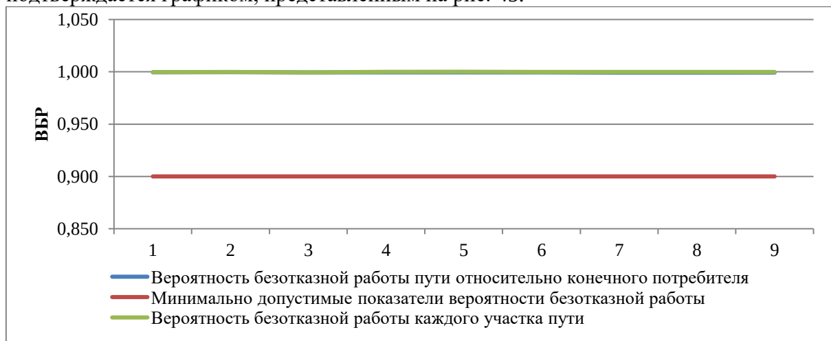
Рисунок 41. ВБР относительно участка тепловой сети от камеры «Вывод Котельная № 17» до потребителя «Пединститут, столовая»
