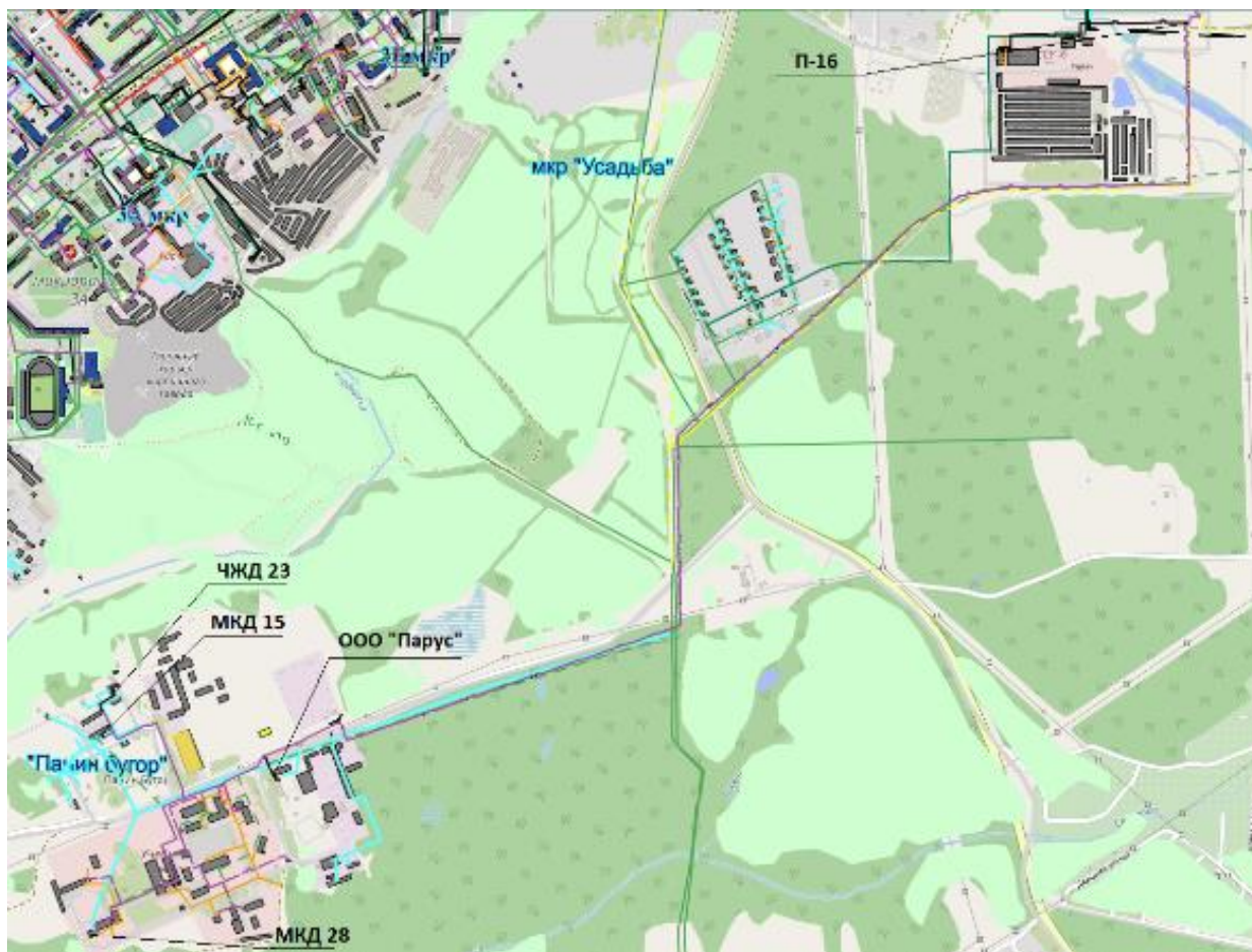
Рисунок 16. Действующая схема подключения мкр. «Панин бугор» от П-16
