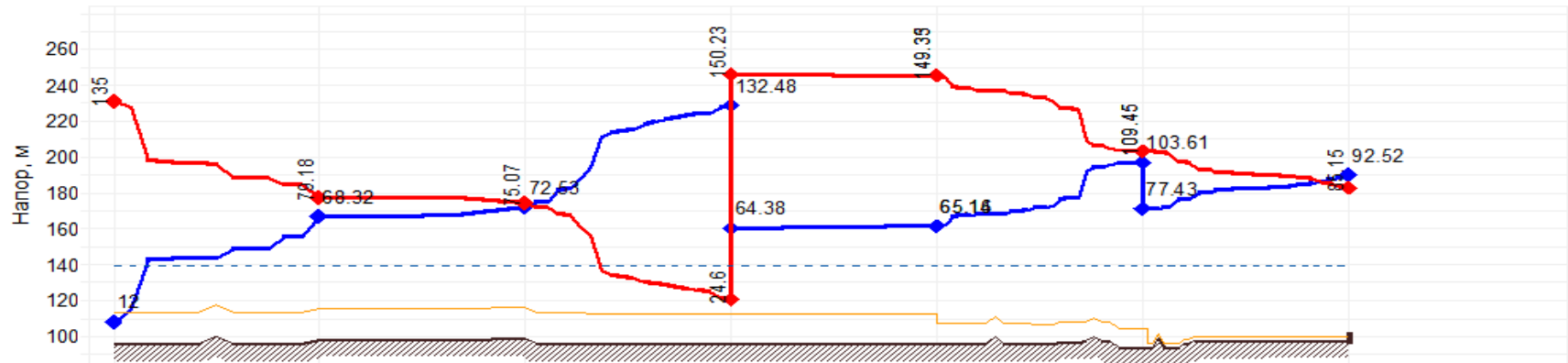
Пьезометрический график от «Тобольская ТЭЦ» до «Драмтеатр»
