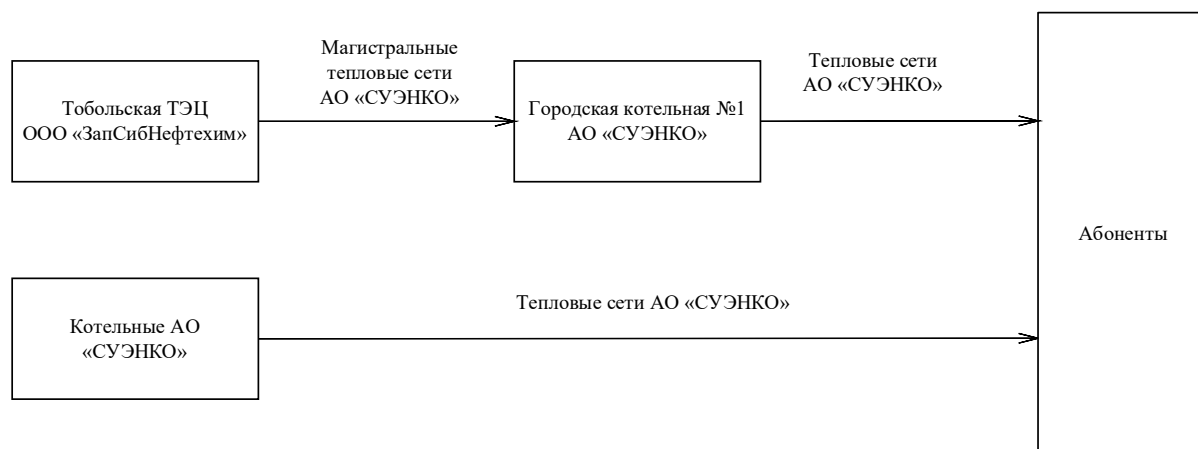
Рисунок 2. Принципиальная схема теплоснабжения города Тобольска
