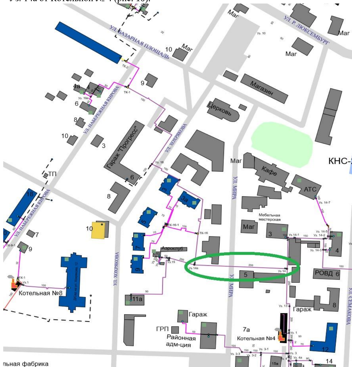
Рисунок 10. Пример моделирования аварийной ситуации на участке тепловой сети Уз. 14 – Уз. 14а от Котельной № 4
