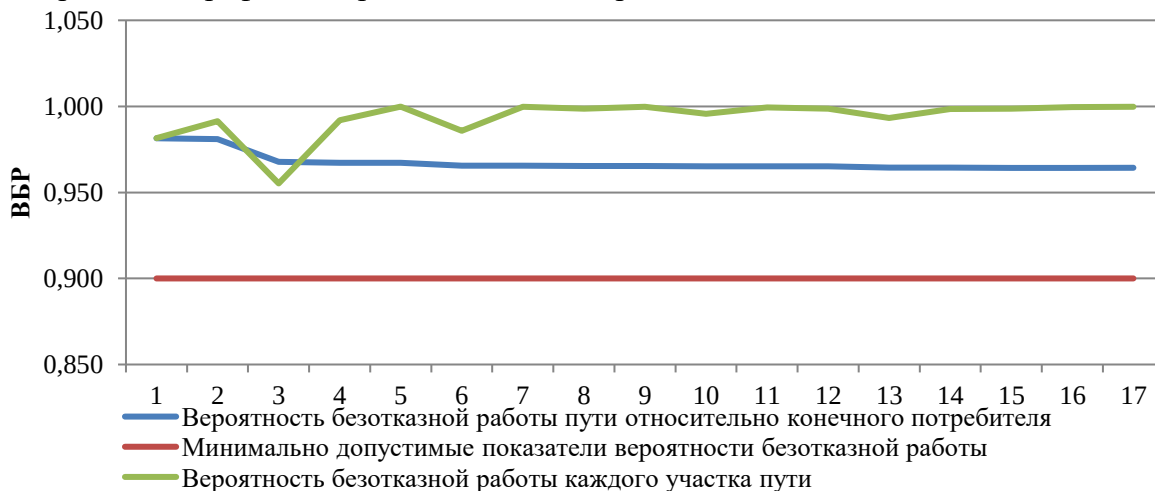
Рисунок 33. ВБР относительно участка тепловой сети от камеры «Вывод - Котельная № 10» до потребителя по ул. Декабристов, 40
