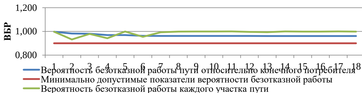
Рисунок 65. ВБР относительно участка тепловой сети от камеры «Вывод - Котельная № 9» до потребителя по ул. Заводская, 11
