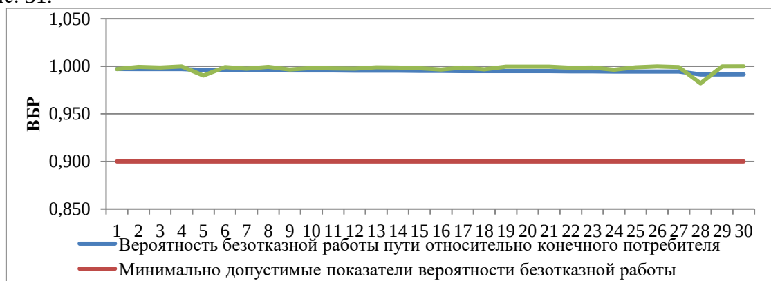
Рисунок 27. ВБР относительно участка тепловой сети от камеры «Вывод - Котельная № 5» до потребителя по ул. Семакова, 58
