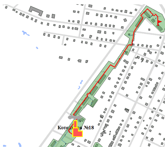
Рисунок 42. Трассировка участка тепловой сети от камеры «Вывод - Котельная № 18» до потребителя по ул. Ленина, 200
