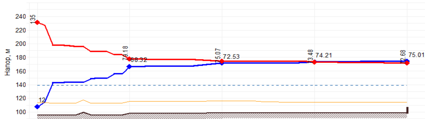
Пьезометрический график от «Тобольская ТЭЦ» до «Произв. к-с, тепл. ст-ка, СММ»
