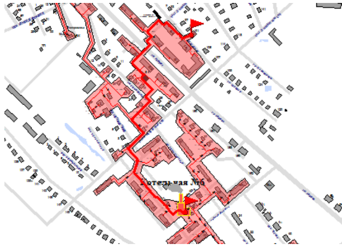
Рисунок 28. Трассировка участка тепловой сети от камеры «Вывод Котельная № 6» до потребителя по ул. Зеленая, 101
