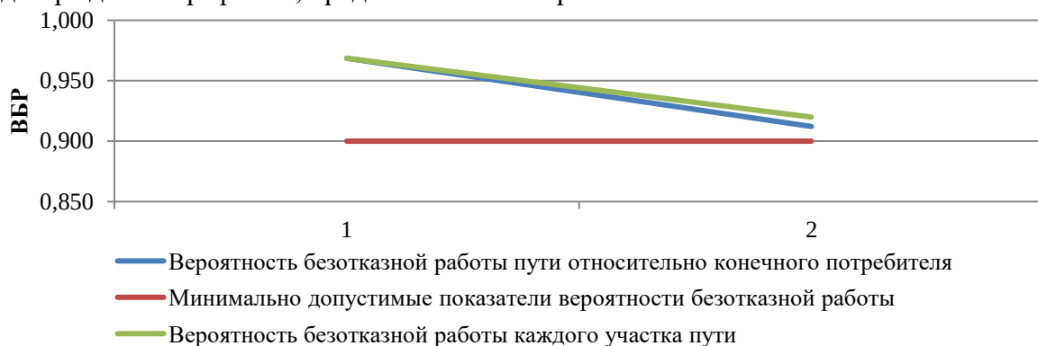
Рисунок 37. ВБР относительно участка тепловой сети от камеры «Вывод -Котельная № 13» до потребителя по ул. 4-я Трудовая, 39
