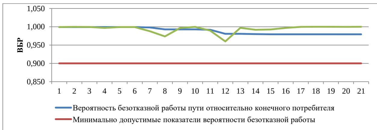
Рисунок 25. ВБР относительно участка тепловой сети от камеры «Котельная № 4» до потребителя «Детский сад № 12»
