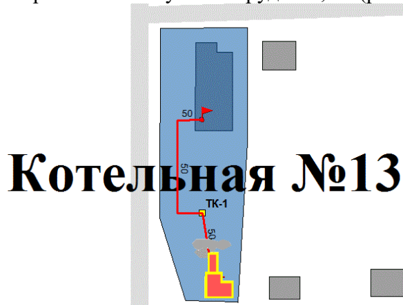
Рисунок 36. Трассировка участка тепловой сети от камеры «Вывод - Котельная № 13» до потребителя по ул. 4-я Трудовая, 39
