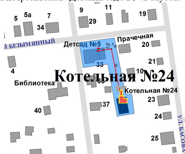
Рисунок 44. Трассировка участка тепловой сети от камеры «Вывод - Котельная № 24» до потребителя «Детский сад № 5 «Голубок»
