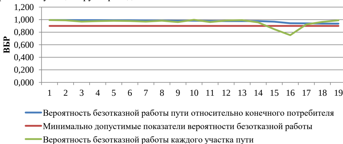
Рисунок 61. ВБР относительно ТК участка тепловой сети от камеры «Вывод - Котельная № 15» до потребителя по ул. Левобережная, 48
