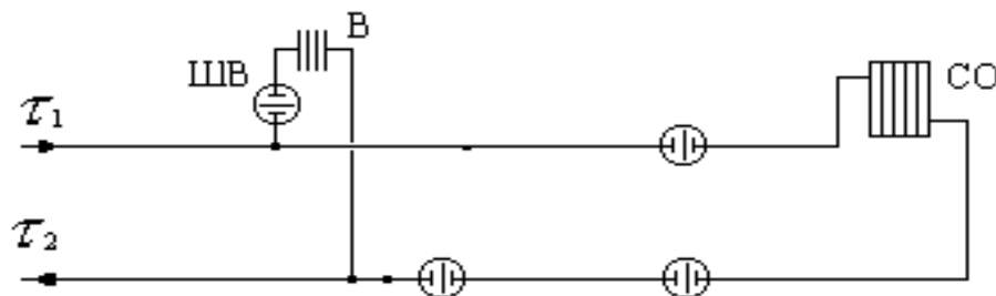
Рисунок 3. Схема «Потребитель с непосредственным присоединением СО»
