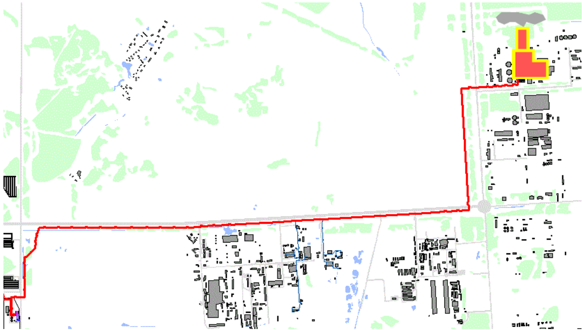
Рисунок 22. Трассировка тепловой сети от Тобольской ТЭЦ до ГК-1
