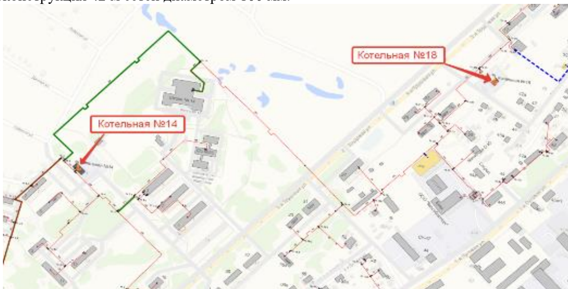
Рисунок 15. Перераспределение нагрузки между котельными № 14 и № 18
