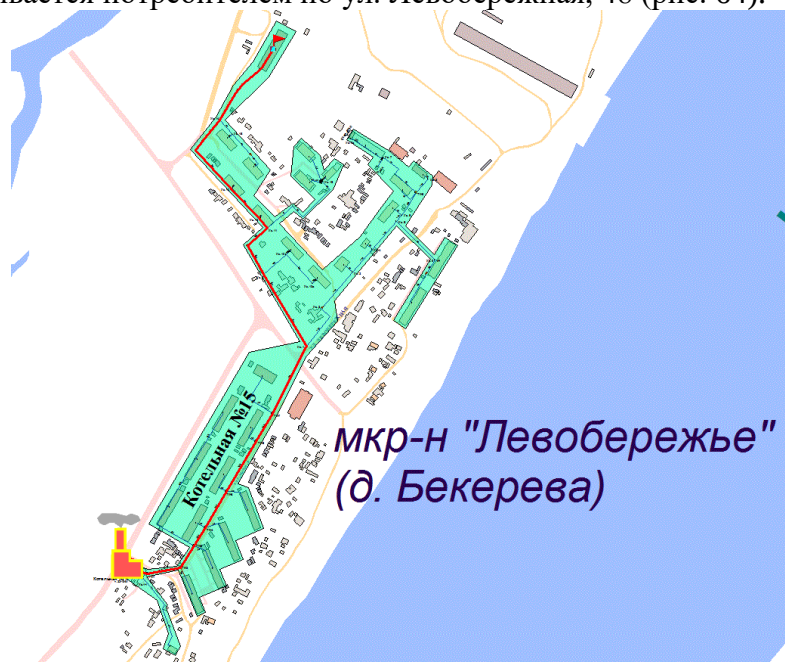
Рисунок 60. Трассировка участка тепловой сети от камеры «Вывод - Котельная № 15» до потребителя по ул. Левобережная, 48
