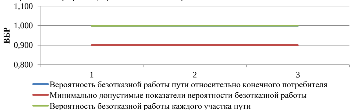
Рисунок 45. ВБР относительно участка тепловой сети от камеры «Вывод - Котельная № 24» до потребителя «Детский сад № 5 «Голубок»
