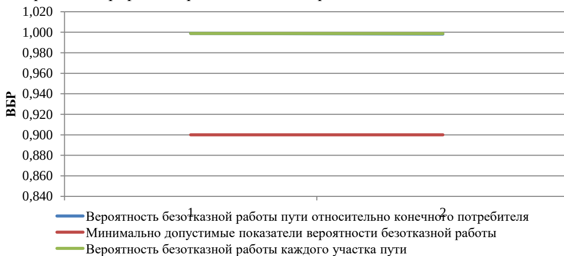
Рисунок 71. ВБР относительно участка тепловой сети от камеры «Вывод - Котельная № 28» до потребителя «Проходная МЧС»
