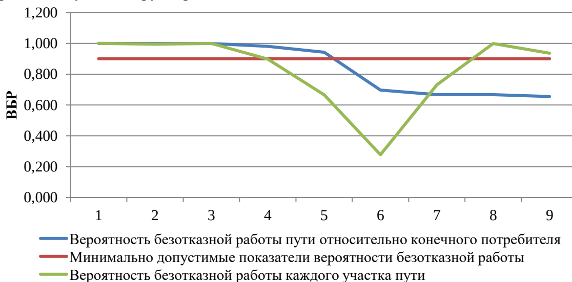
Рисунок 57. ВБР относительно участка тепловой сети от камеры «Вывод - Котельная № 22» до потребителя «Эстетический центр»
