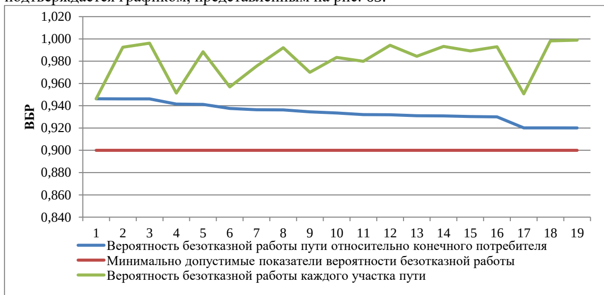
Рисунок 59. ВБР относительно участка тепловой сети от камеры «Вывод - Котельная № 16» до потребителя ул. Крупской, 16, Южакова Г.Г.
