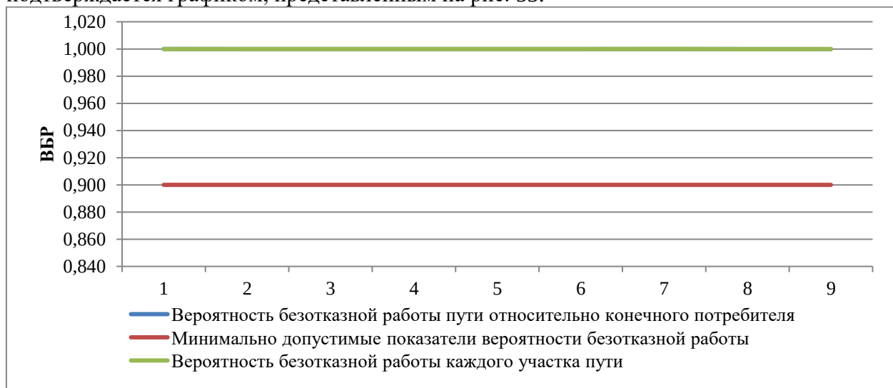
Рисунок 49. ВБР относительно участка тепловой сети от камеры «Вывод - Котельная № 29» до потребителя «Базарная площадь, магазин»
