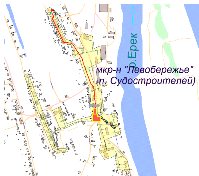
Рисунок 62. Трассировка участка тепловой сети от камеры «Вывод - Котельная № 19» до потребителя по ул. Калинина, 5
