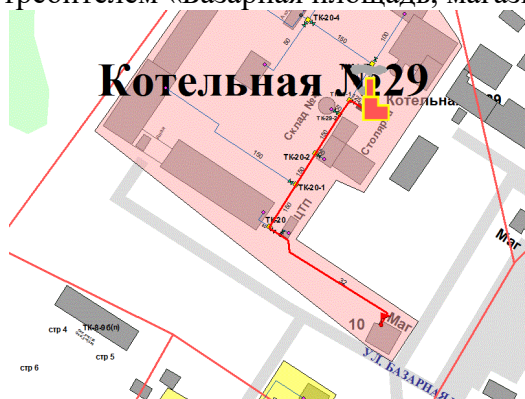
Рисунок 48. Трассировка участка тепловой сети от камеры «Вывод - Котельная № 29» до потребителя «Базарная площадь, магазин»
