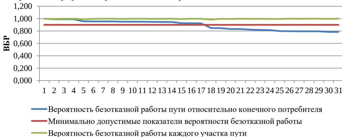
Рисунок 53. ВБР относительно участка тепловой сети от камеры «Вывод - Котельная № 3» до потребителя по ул. Верхнефилатовская, 1
