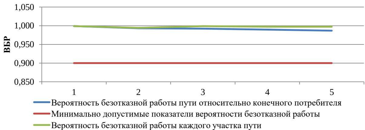
Рисунок 51. ВБР относительно участка тепловой сети от камеры «Вывод - Котельная № 31» до потребителя «Школа № 1, мастерские»
