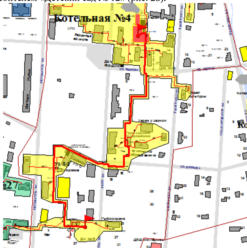
Рисунок 24. Трассировка тепловой сети от камеры «Котельная № 4» до потребителя «Детский сад № 12»
