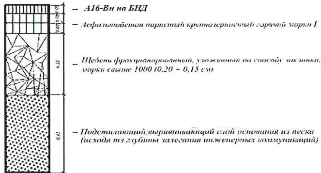
Тип 1. Конструкция дорожной одежды на проезжей части автомобильной дороги (Группа А)
