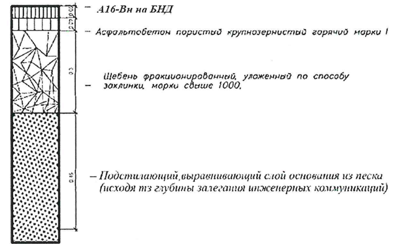
Тип 10. Конструкция дорожной одежды на проезжей части и стоянках, расположенных на территориях, не относящихся к автомобильным дорогам и проездам
