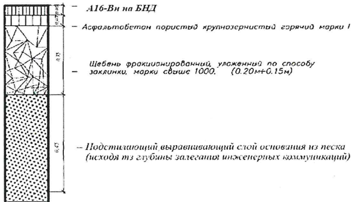
Тип 2. Конструкция дорожной одежды на проезжей части автомобильных дорог (Группа Б)
