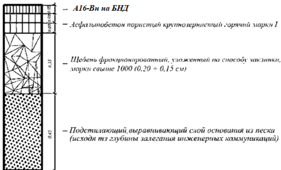
Тип 1. Конструкция дорожной одежды на проезжей части автомобильной дороги (Группа А)
