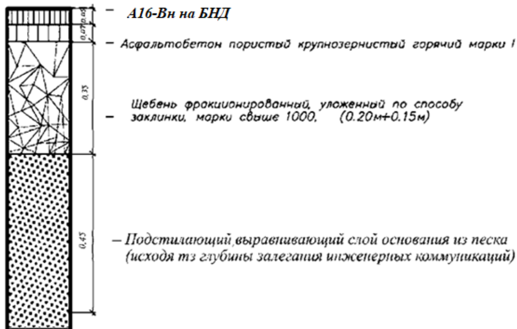
Тип 2. Конструкция дорожной одежды на проезжей части автомобильных дорог (Группа Б)
